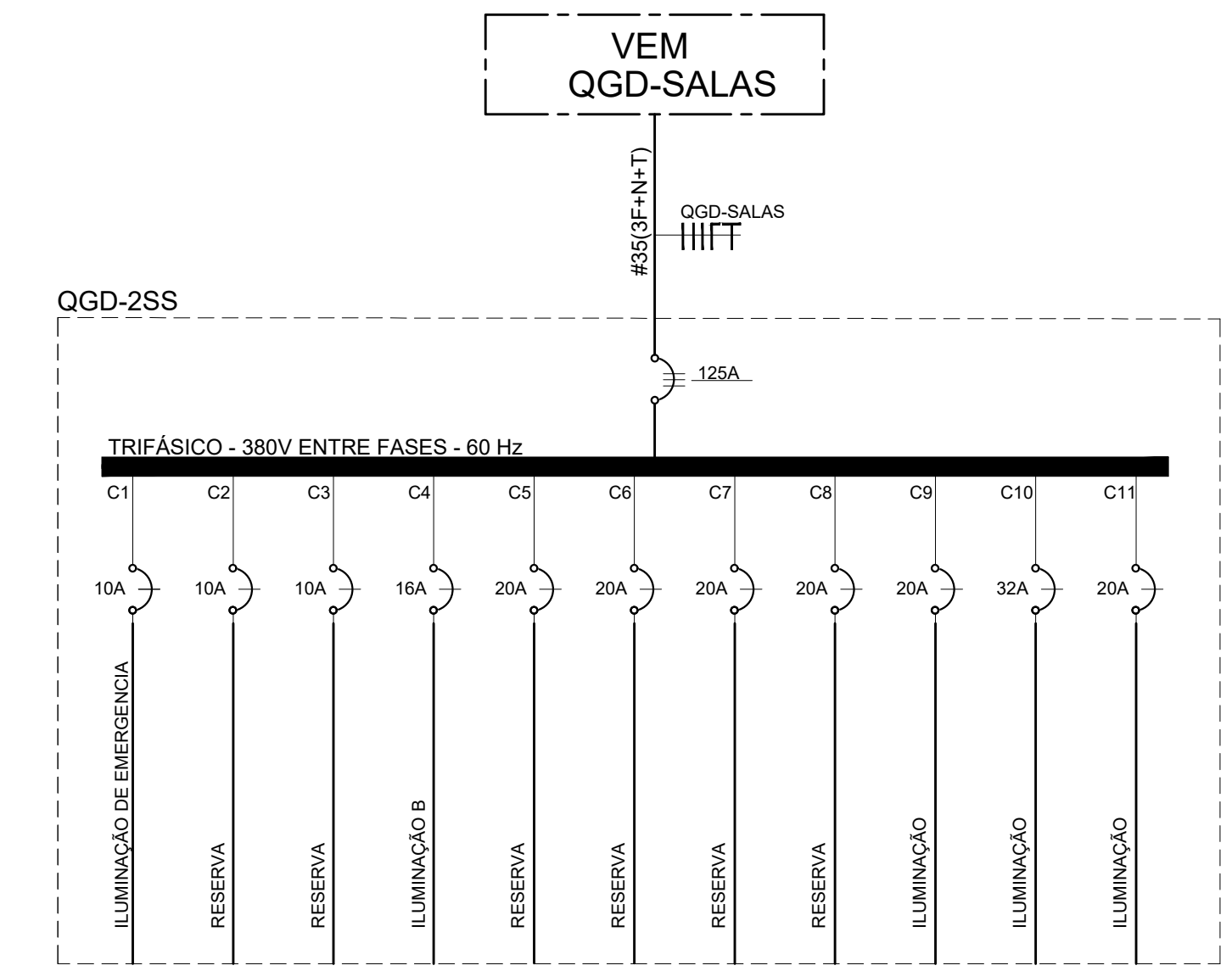
DIAGRAMA UNIFILAR QGD 2º SUBSOLO
